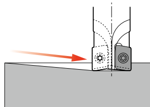
斜向進刀
